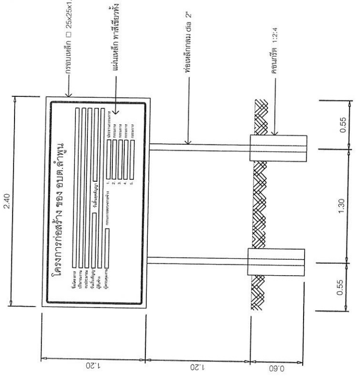
แปลน 1:25
